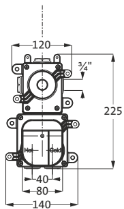
Rohbauset für Thermostate für 1 Verbraucher, LA433200
