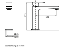
LARIMAR E1 Waschtischmischer M-Size 130 ohne Ablaufgarnitur, chrom
