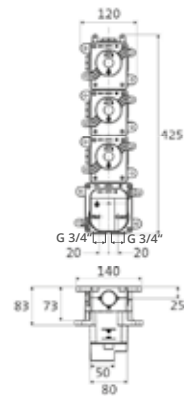
Rohbauset für Thermostat mit 3 Absperrventilen chrom, LA433100
