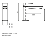
LARIMAR E1 Waschtischmischer S-Size 120 ohne Ablaufgarnitur, chrom
