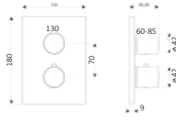
Unterputz-Feinbauset für Wannenfüll- /Brausethermostat eckige Rosette, eigensicher gegen Rückfließen, chrom, LA434220500
