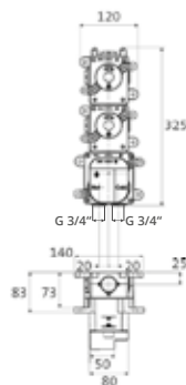
Rohbauset für Thermostat mit 2 Absperrventilen chrom, LA433000
