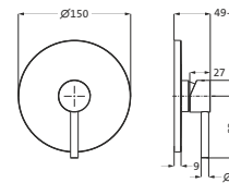
A2 UP-Brause-Fertigmontageset, Blende rund, chrom, LA404320500
