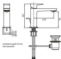
LARIMAR E1 Waschtischmischer S-Size 120 mit Ablaufgarnitur, chrom
