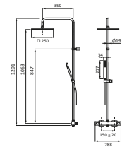
LARIMAR E1 Duschsystem mit Thermostat, Slim-Kopfbrause 250x250 mm, Stabh., chrom LA452710500
