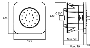
LARIMAR E1 Seitenbrause schwenkbar, inkl. Unterputzkörper, chrom LA452870500
