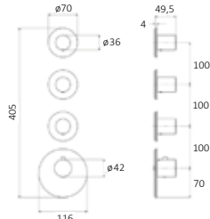
Unterputz Feinbauset mit 3 Absperrventilen für Brausethermostat, eigensicher gegen Rückfließen, mit 4 Einzelrosetten, chrom, LA433120500
