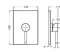
A2 UP-Brause-Fertigmontageset Blende eckig, chrom, LA404321500
