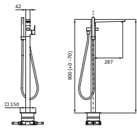
LARIMAR E1 Wannen-Standarmatur ohne Einbaubox, chrom LA405450500
