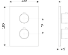
Unterputz-Feinbauset für Brausethermostat eckige Rosette, eigensicher gegen Rückfließen, chrom, LA434120500
