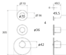
Unterputz Feinbauset mit 2 Absperrventilen für Brausethermostat, eigensicher gegen Rückfließen, mit 3 Einzelrosetten, chrom, LA433020500
