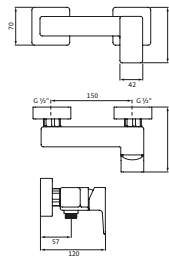
LARIMAR E1 AP-Brausemischer chrom LA405300500
