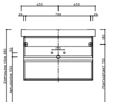
Unterschrank Breite 840 mm, 2 Auszüge LA08064...
