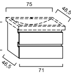
Unterschrank Breite 710 mm, 2 Auszüge, LA080553...
