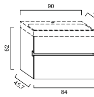
LARIMAR 3 WTU, 839/620/457 cm, 1 Lade, 1 Auszug zu M100 LA086104
