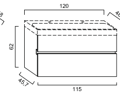
LARIMAR 3 WTU, 1149/620/457 cm, 1 Lade, 1 Auszug zu M100 LA086105
