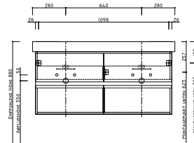
Unterschrank Breite 1150 mm, 4 Auszüge LA08064...
