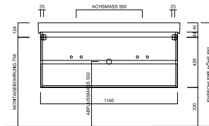
Waschtisch-Unterschrank LA080555..., Abb. wenn Armatur links ist
