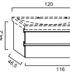
Unterschrank Breite 1160 mm, 2 Auszüge, LA080555...
