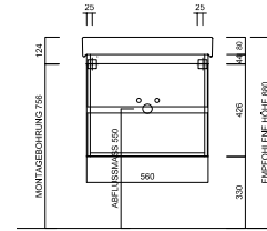
Waschtisch-Unterschrank LA080552...
