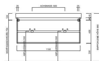
Waschtisch-Unterschrank LA080556...
