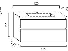
LARIMAR 3 WTU, 1 Lade, 1 Auszug, 1189/620/477 cm, zu K3 LA086035
