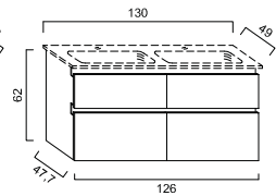
LARIMAR 3 WTU, 1 Lade, 1 Auszug, 1259/620/477 cm, zu K3 LA086036
