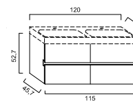
Unterschrank Breite 1150 mm, 4 Auszüge, LA08064...
