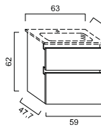
LARIMAR 3 WTU, 1 Lade, 1 Auszug, 589/620/477 cm, zu K3 LA086032
