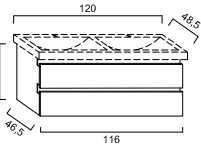
Unterschrank Breite 1160 mm, 2 Auszüge, LA080556...
