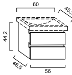
Unterschrank Breite 560 mm, 2 Auszüge, LA080552...
