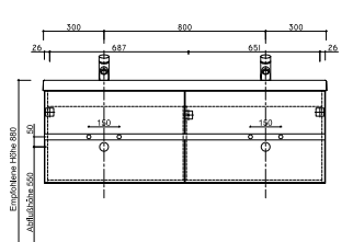
Waschtisch Cassetta Breite 1400 mm, Tiefe 450 mm mit Unterschrank Breite 1390 mm, 4 Auszüge, LA08077...
