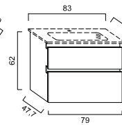
LARIMAR 3 WTU, 1 Lade, 1 Auszug, 789/620/477 cm, zu K3 LA086033
