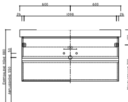
Unterschrank Breite 1150 mm, 4 Auszüge LA08064...
