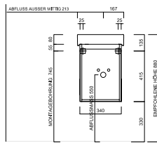
Handwaschbecken-Unterschrank LA080551..., LA080550...
