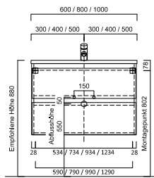
Waschtischunterbau Tiefe 538 mm, Breite 590/790/990 mm
