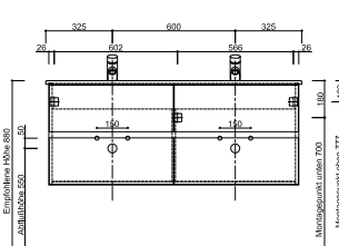
Waschtisch „Cult“ Breite 1250 mm, Tiefe 470 mm mit Unterschrank Breite 1220 mm 4 Auszüge, LA08076...
