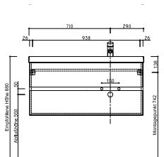
Waschtisch „Campus“ Breite 1000 mm, Tiefe 450 mm mit Unterschrank Breite 990 mm, 2 Auszüge, LA08075...
