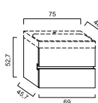
Unterschrank Breite 690 mm, 2 Auszüge, LA08064...
