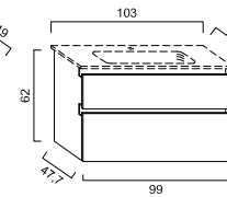
LARIMAR 3 WTU, 1 Lade, 1 Auszug, 989/620/477 cm, zu K3 LA086034
