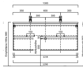
Waschtischunterbau für Trogwaschtisch Tiefe 538 mm, Breite 1290 mm
