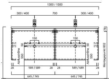
Doppelwaschtischunterbau Tiefe 538 mm, Breite 1290/1490 mm
